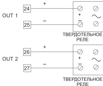
Рис. 10 ПРОВОДКА ВЫХОДА ПРИВОДА SSR
